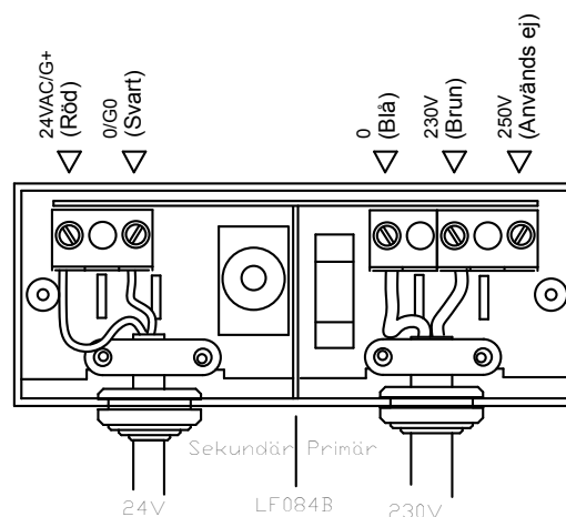
Mått och inkopplingar för installation av LF084B. Ledare kopplas in enligt färgangivelsen.
