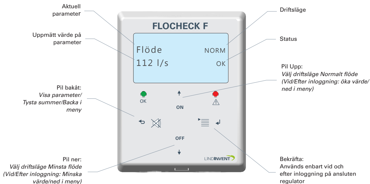
Knappar och display på dragbänksvakt FLOCHECK F.
