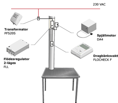
Dragbänk med Flocheck F och övriga komponenter för flödesstyrning.
