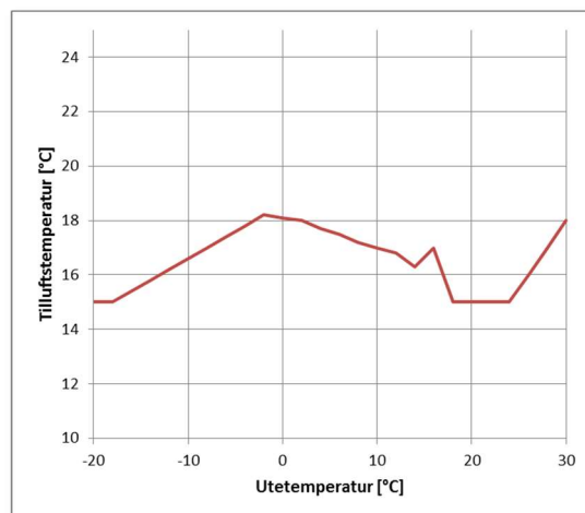
Exempel på tilluftstemperatur för aggregat med roterande värmeväxlare och temperaturoptimering (dimensionerande utetemperatur 25°C).
