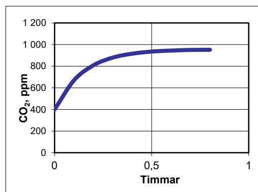
Koldioxidhalt i ett gym med 10 personer, luftflöde 300 l/s. CO 2 -avgivning 60 l/h och person, omblandande ventilation.
