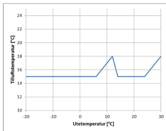
Exempel på tilluftstemperatur för aggregat med vätskekopplade batterier och temperaturoptimering (dimensionerande utetemperatur 25°C).
