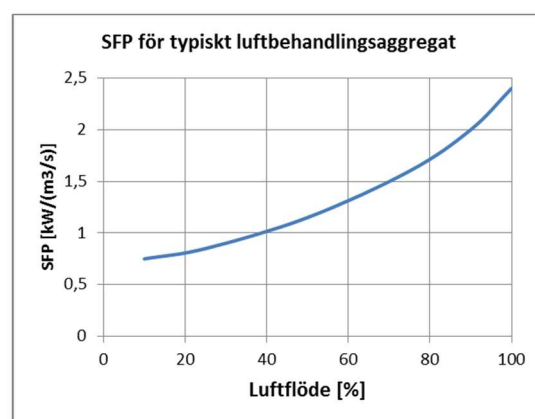
SFP för typiskt luftbehandlings aggregat.
