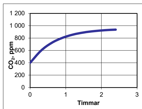
Koldioxidhalt i enpersons kontor med luftflöde 10 l/s. CO 2 -avgivning 20 l/h, omblandande ventilation.
